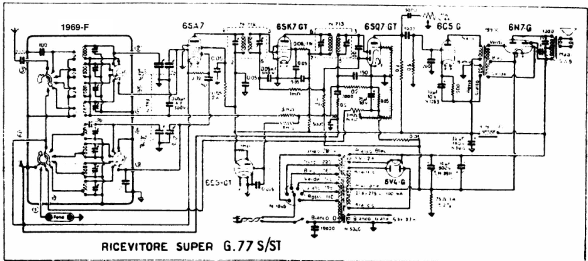
Lo schema elettrico.
